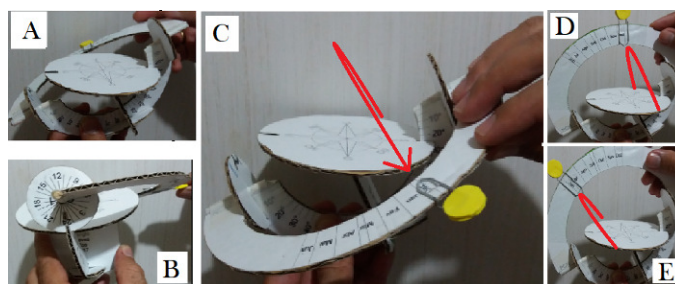
Figura 11: Simulando o Movimento Aparente do Sol com o SUMAS.
