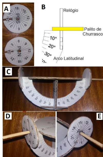
Figura 6: Fixação dos relógios em ambas nas porções opostas do AL. A= Relógios de 24 horas PCS e PCN. B= Detalhe em perfil do posicionamento do palito de churrasco no AL e no Relógio 24 horas. C= Os relógios PCS e PCN posicionados em ambas as porções do AL. D= Detalhe do relógio PCN posicionado correspondente à direção cardinal Norte. E= Detalhe do relógio PCS posicionado correspondente à direção cardinal Sul.
