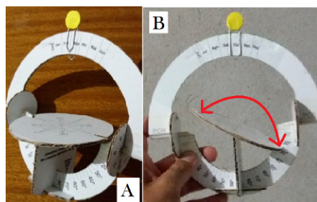
Figura 10: Posição do disco horizontal em detrimento da latitude. A= Simulação do observador na latitude 0^\circ ; B= Simulação do observador na latitude 25^\circ\text{S} .
