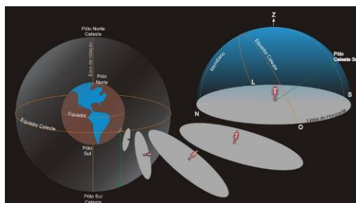
Figura 9: Projeção da posição do observador em detrimento de sua posição terrestre e a esfera celeste (OLIVEIRA FILHO, SARAIVA, 2010).
