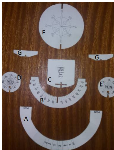
Figura 2: Peças do Simulador Universal do Movimento Aparente do Sol coladas e recortadas em papelão.
