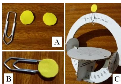
Figura 8: Construção e posicionamento do “Sol” no SUMAS. A= 1 clips e 2 discos amarelos (em EVA); B= Montagem do simulado de Sol; C= Posicionamento do Sol no SUMAS.
